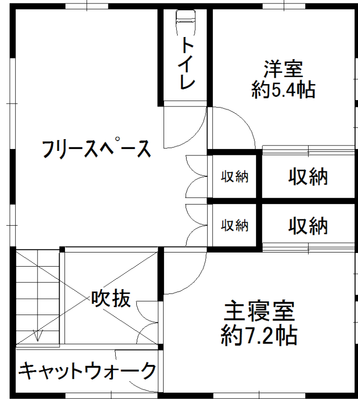
2階平面図
